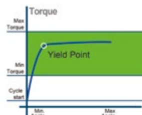
Límite elástico (Análisis de Junta)
