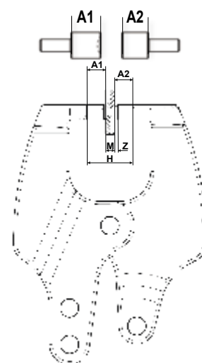
1 set de remache a ras + 1 set ahuecado Z=0
