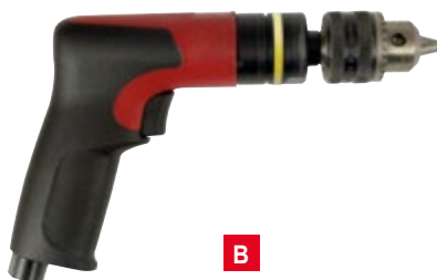
B Serie DR50 500 W (0.68 hp) - 400 a 18500 rpm
