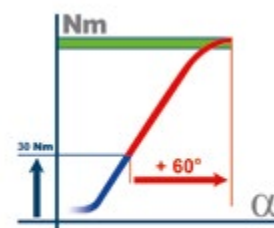
Apriete con toque y ángulo de rotación adicional (par + ángulo)
