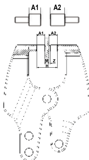
Dos set de remachado a ras
