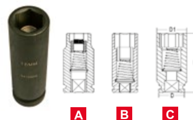
Vaso largo magnético 1/2"
