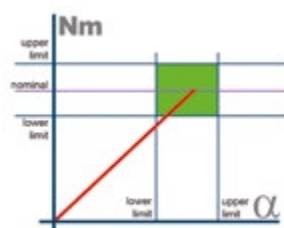
Aprietes dentro de límites de par y ángulo (apriete en una ventana)
