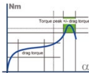
Compensación automática de par prevaeciente
