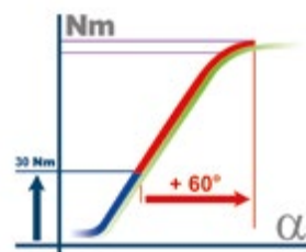
Apriete con par y rotación de ángulo adicional (par + ángulo)
