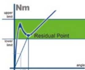
Par Residual (VDI-VDE 2645-3)
